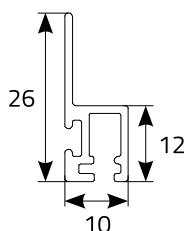
profil dolny „h” (standard)
