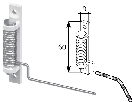
samozamykacz (moskitiera z futryną)
