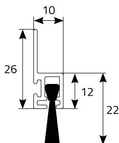
profil dolny "h" (Typ2_H) (konstrukcje z progiem)
