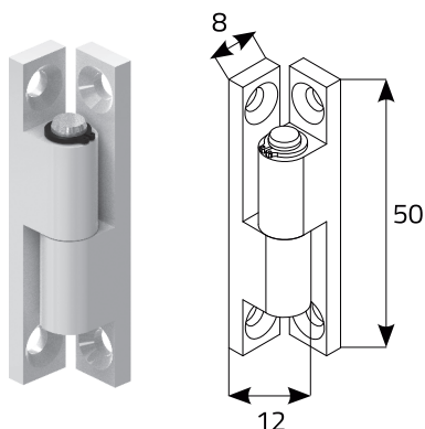
zawias aluminiowy (standard)
