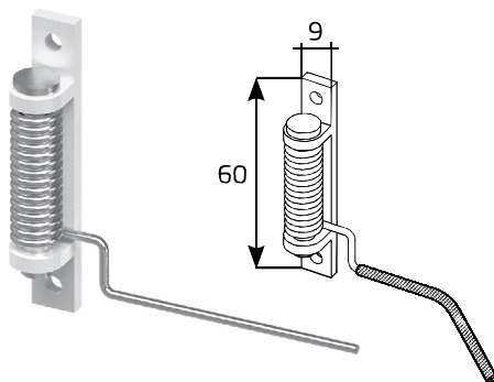
Türschließer (Insektenschutztür mit Rahmen)
